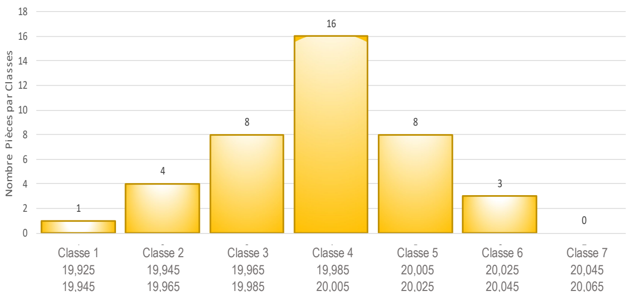
HISTOGRAMME des AXES USINÉS
